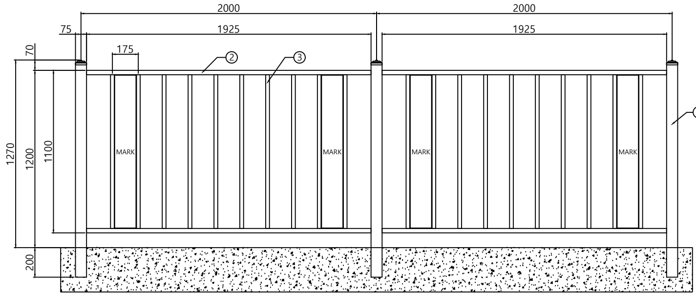
① 정면도
